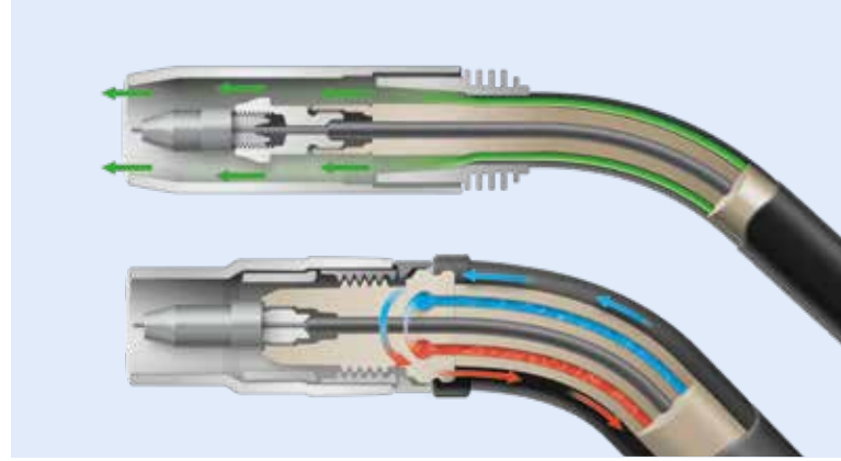
MSG-Brenner: gasgekühlt (oben) und flüssiggekühlt (unten)
